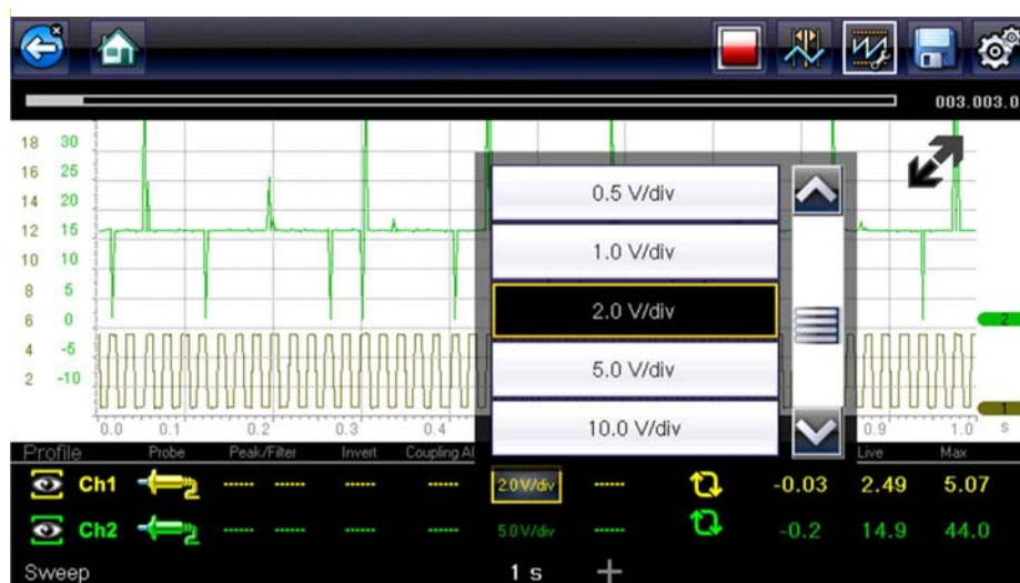
Figura 10-15 Tela do multímetro e osciloscópio definida para Por divisão
